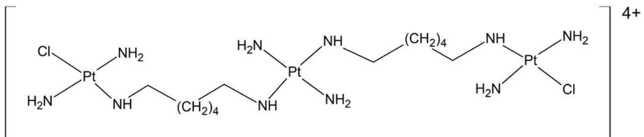
Obr. 7. Štruktúra komplexu BBR3464
