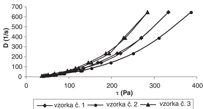
Obr. 4. Tokové krivky vzorky č. 1–3
