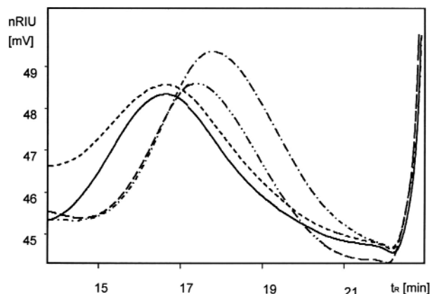
Obr. 1. Chromatogramy vzorků CMC Na šarže 283/2011 sterilizovaných \gamma -zářením (---), \beta -zářením (-·-·-), ethylenoxidem (····) a nesterilizovaných (—)
