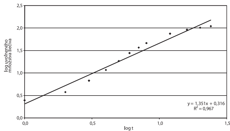
Obr. 10. Príklad D, parametre Korsmejer-Peppasovho modelu spracované z disolučných údajov in vitro
